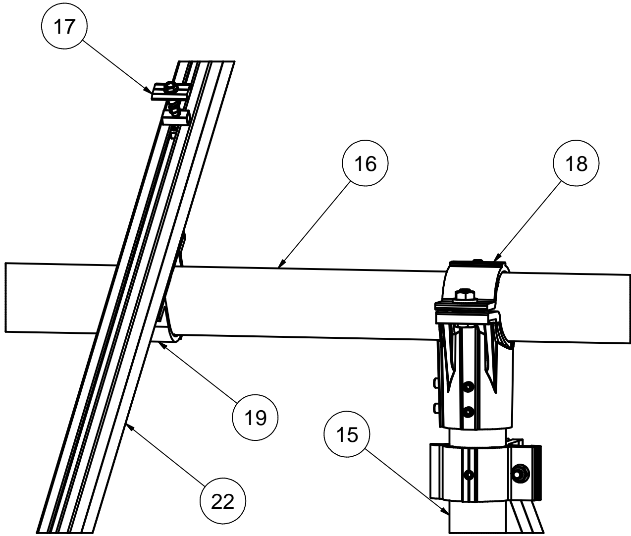
DETAIL A-ALT
