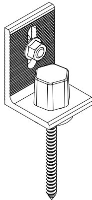
EZ Metal Roof Mount, EZ L-Footer K10082-001
