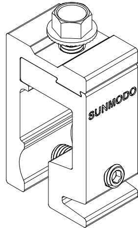
2" EZ STANDING SEAM CLAMP, MINI K50210-002
